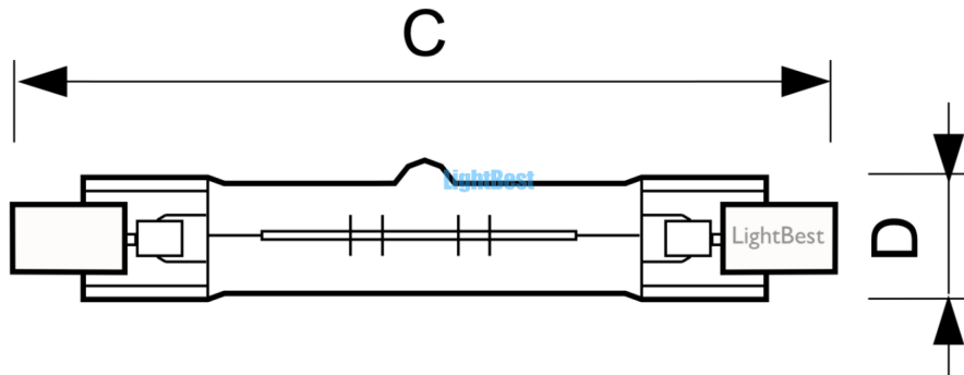
Лампа галогенная LightBest LBH 9067 150W 220V R7s 118mm
