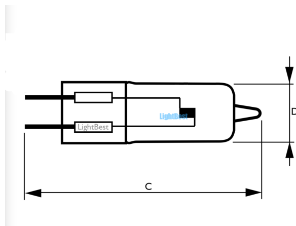
Лампа галогенная LightBest LBH 9095 100W 24V G6.35
