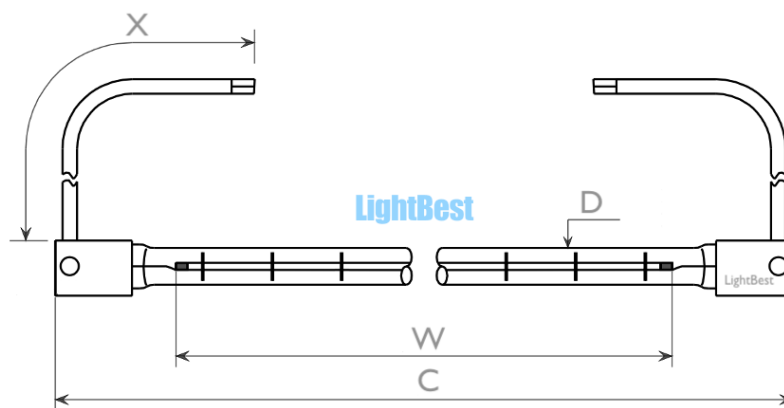
Лампа инфракрасная LightBest IRK 9043 1000W 400V SK15 RU355
